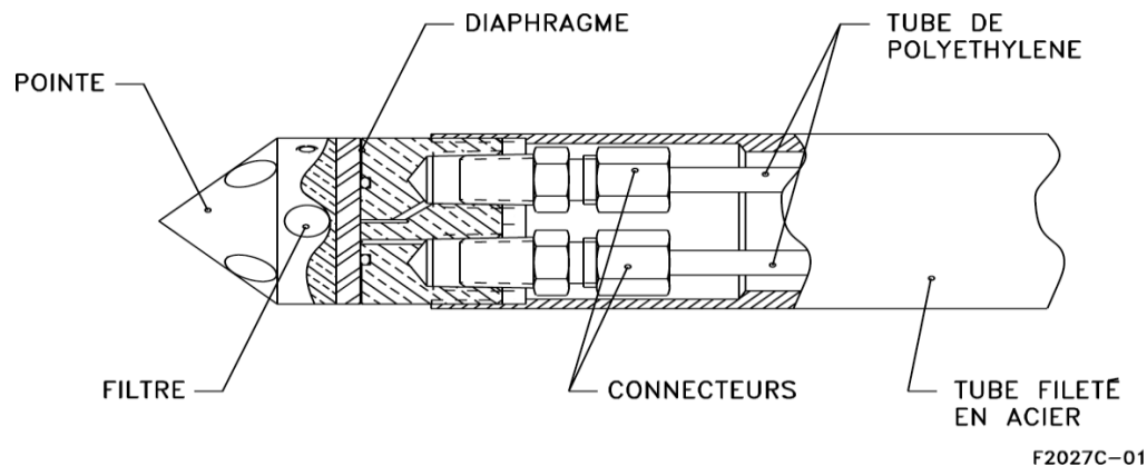
FIGURE 1 : Schéma du piézomètre pneumatique modèle FPC-2
