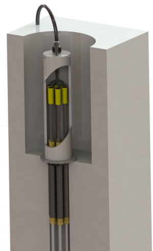
Tête de référence BOREX-E avec multiconducteur
